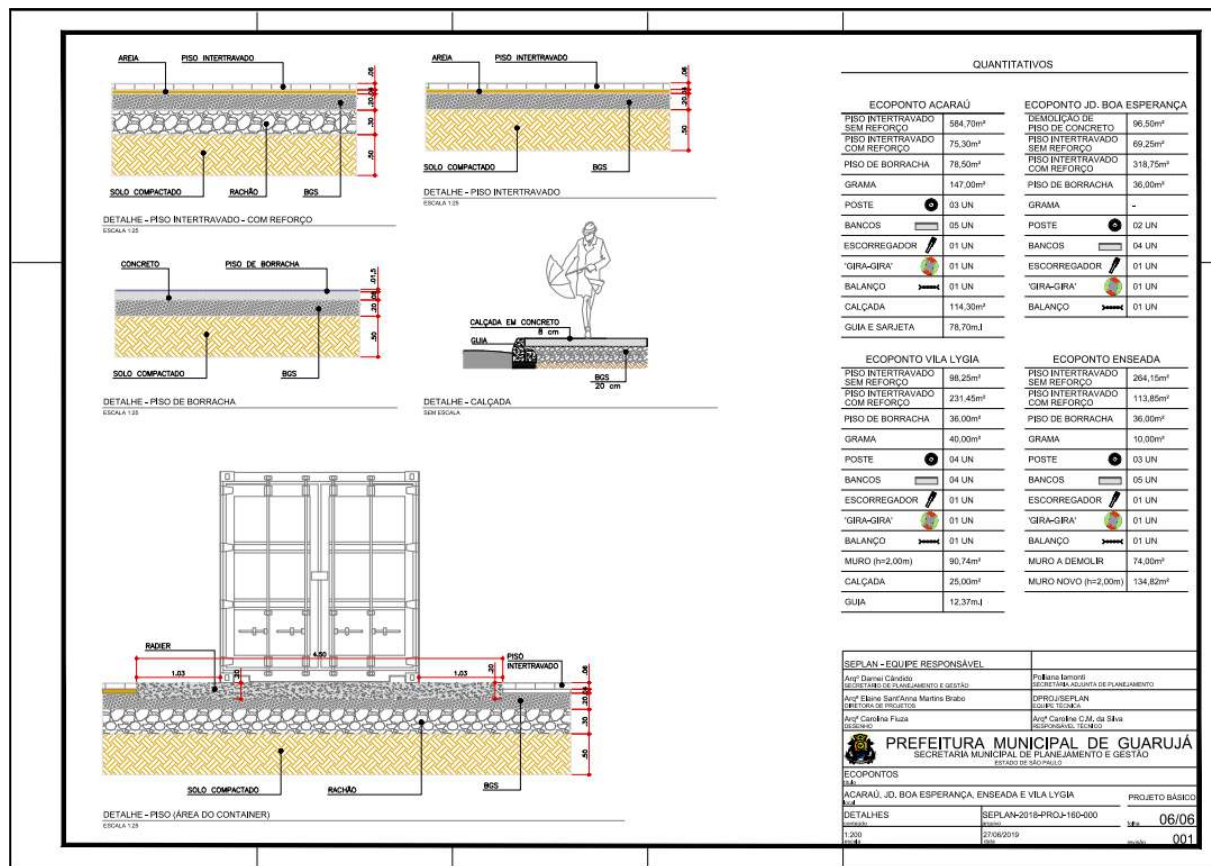
Figura 27: Especificações técnicas, detalhes e quantitativos dos Ecopontos.
