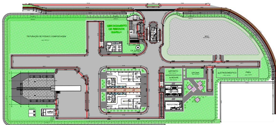
Figura 25: Implantação Centro de Gerenciamento de Resíduos Sólidos.
